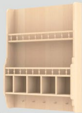
编号：SG100 颜色：榉木水性木蜡油 尺寸：高1200*宽900/1000*深200mm
